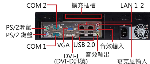
後視圖
